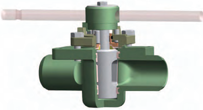
FIG. P260N BW 316/316
